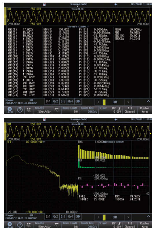
高調波解析結果のリスト表示(上)およびバーグラフ、FFT表示(下)
