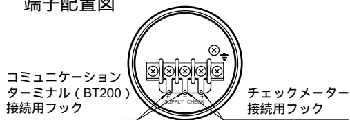
端子配置図
