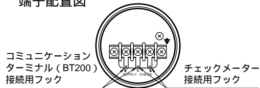
端子配置図
